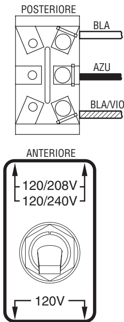
INTERRUPTOR SERLECTOR DE VOLTAJE
